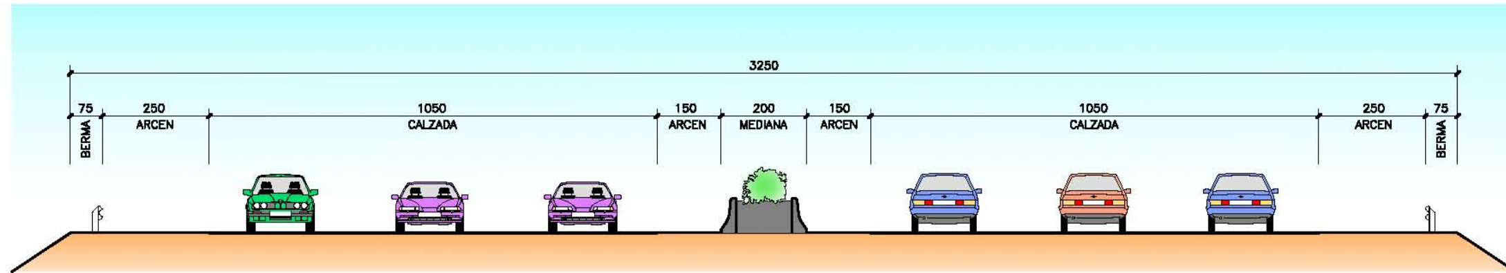
SECCION 10 ESCALA 1/80 COTAS EN cm
