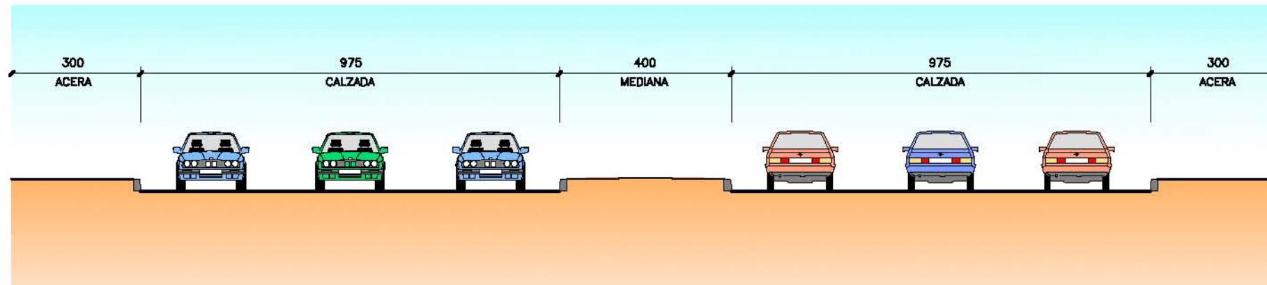
SECCION 15 ESCALA 1/60 COTAS EN cm
