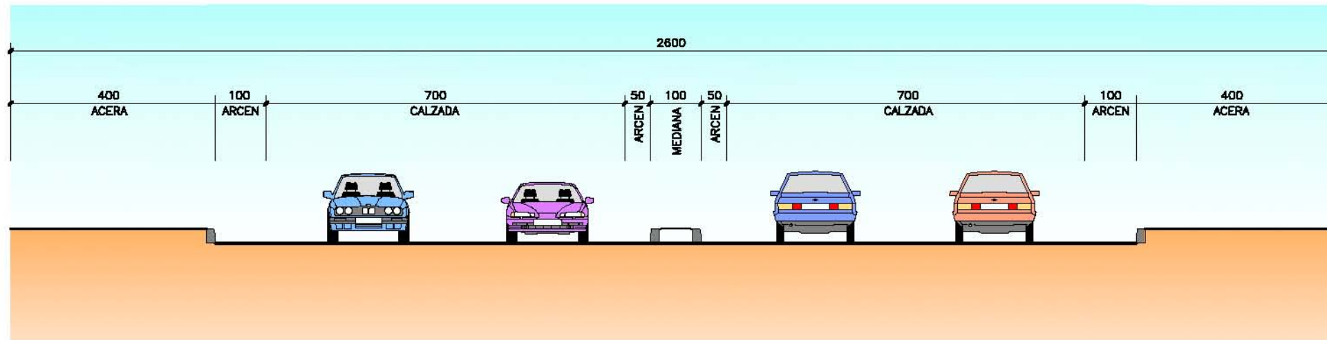
SECCION 12 ESCALA 1/50 COTAS EN cm
