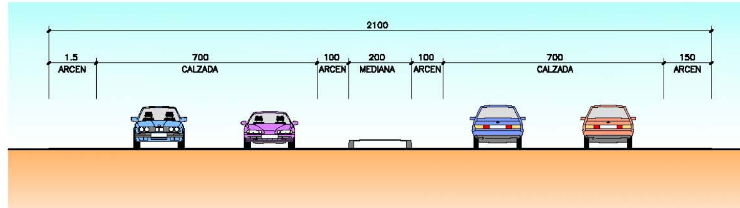
SECCION 6 ESCALA 1/60 COTAS EN cm
