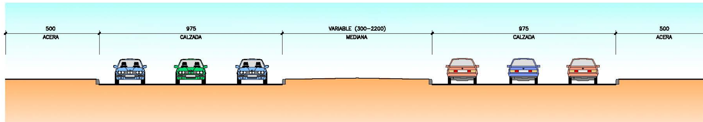
SECCION 16 ESCALA 1/60 COTAS EN cm
