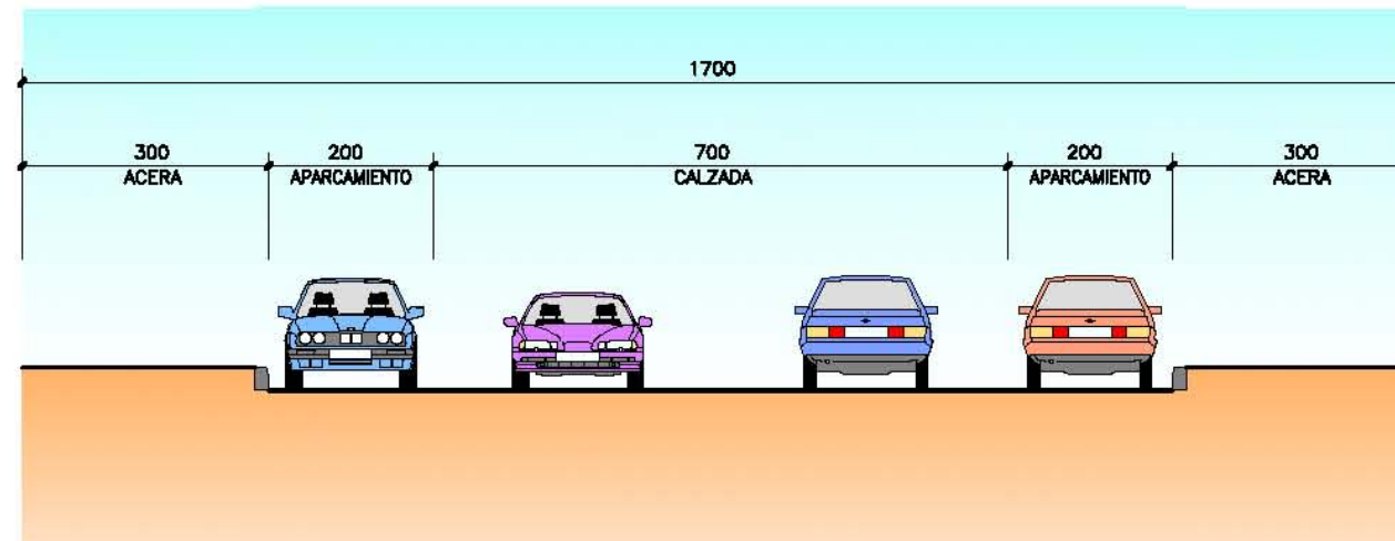
SECCION 13 ESCALA 1/60 COTAS EN cm
