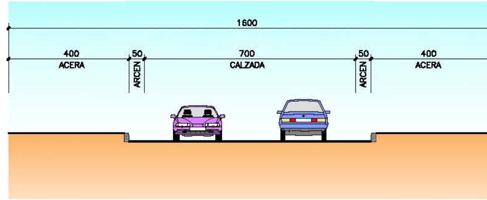
SECCION 5 ESCALA 1/80 COTAS EN cm
