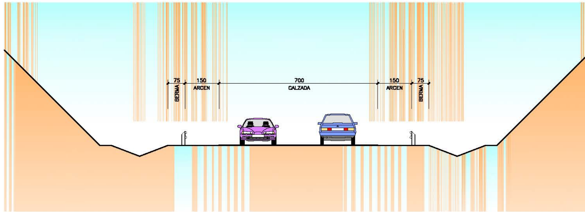
SECCION 3 ESCALA 1/50 COTAS EN cm
