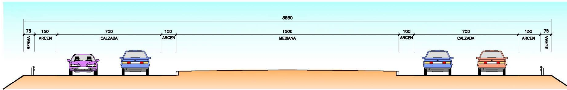
SECCION 8 ESCALA 1/60 COTAS EN cm
