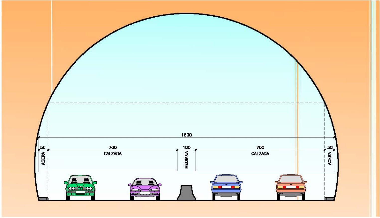
SECCION 2 ESCALA 1/50 COTAS EN cm
