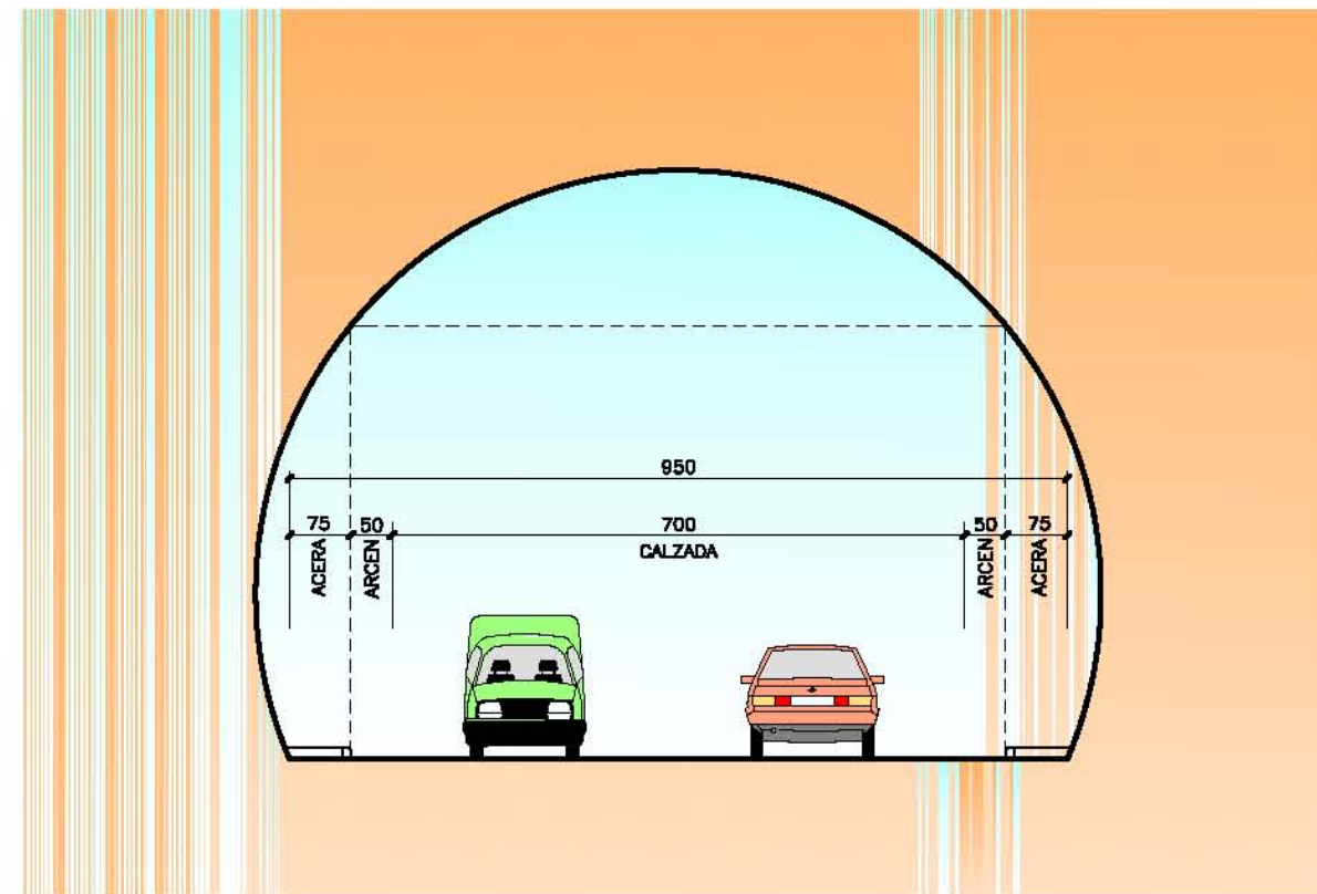
SECCION 4 ESCALA 1/50 COTAS EN cm
