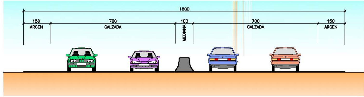
SECCION 1 ESCALA 1/50 COTAS EN cm
