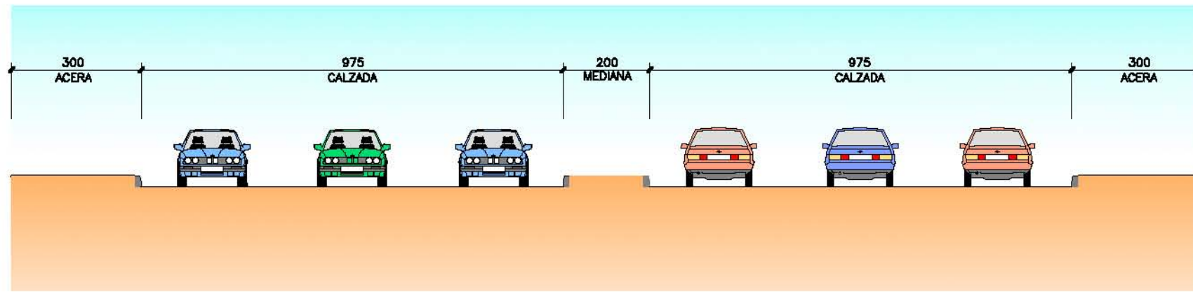
SECCION 14 ESCALA 1/60 COTAS EN cm
