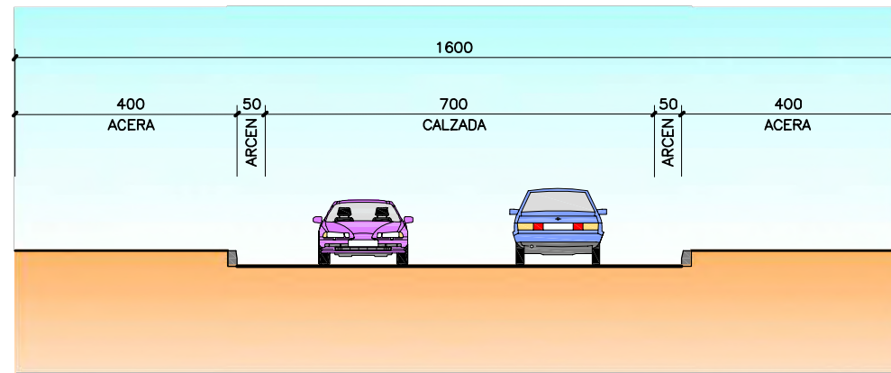
SECCION 5 ESCALA 1/60 COTAS EN cm
