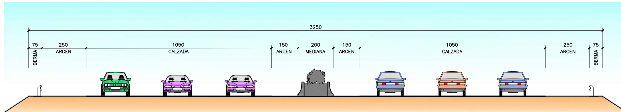
SECCION 10 ESCALA 1/60 COTAS EN cm
