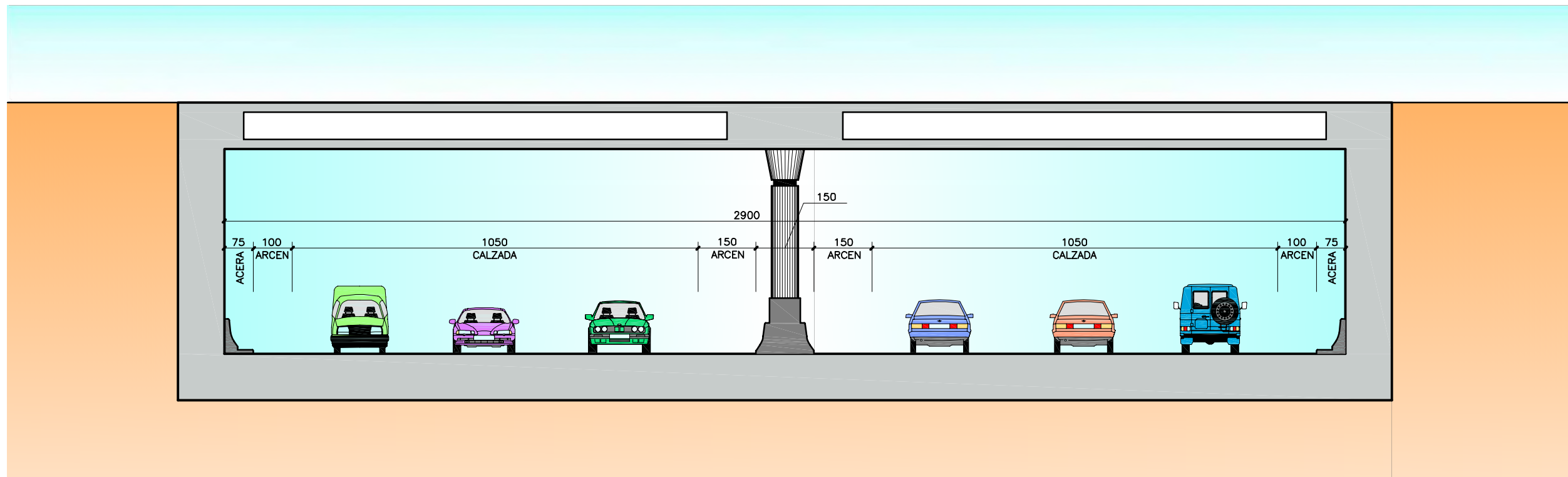
SECCION 11 ESCALA 1/60 COTAS EN cm
