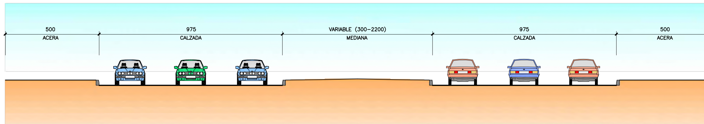
SECCION 16 ESCALA 1/60 COTAS EN cm
