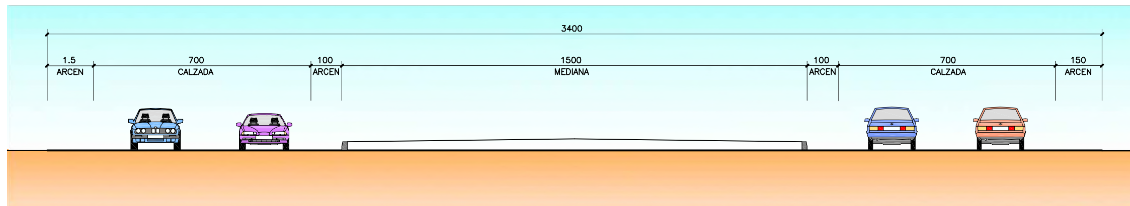
SECCION 7 ESCALA 1/60 COTAS EN cm
