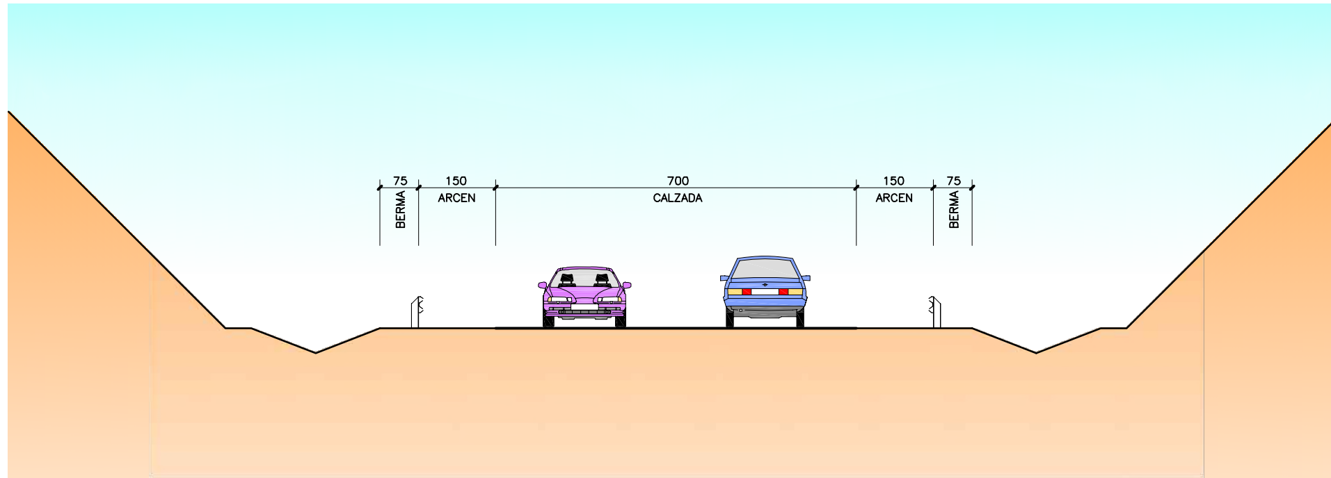
SECCION 3 ESCALA 1/50 COTAS EN cm
